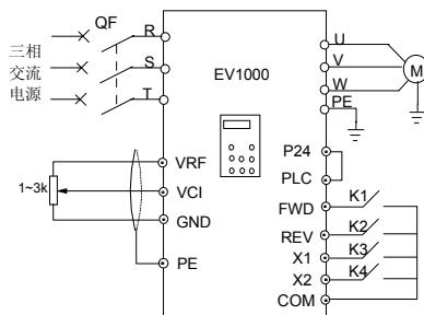
图 5-57 两地控制硬件接线图
