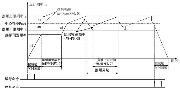
图 5-36 摆频示意图
