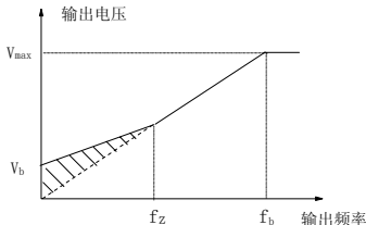
图 5-3 转矩提升（提升量为阴影部分）
