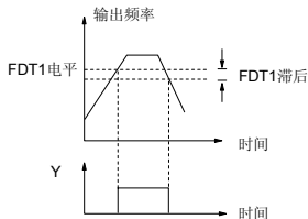
图 5-47 频率水平检测示意图
